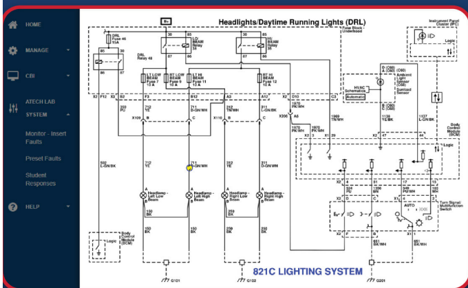
Wiring schematics
